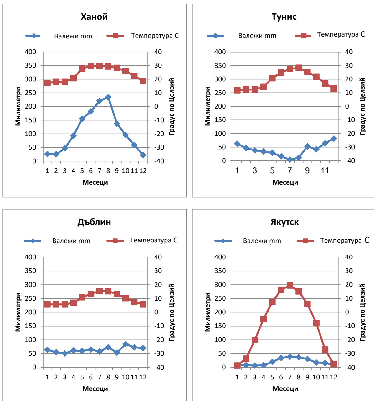
Фигура 1: Климатичните диаграми се състоят от диаграма на валежите и диаграма на температурата. Вляво са показани валежите в милиметри, а вдясно - температурата в градуси по Целзий. Диаграмите показват средните стойности на валежите и температурата от януари до декември.
